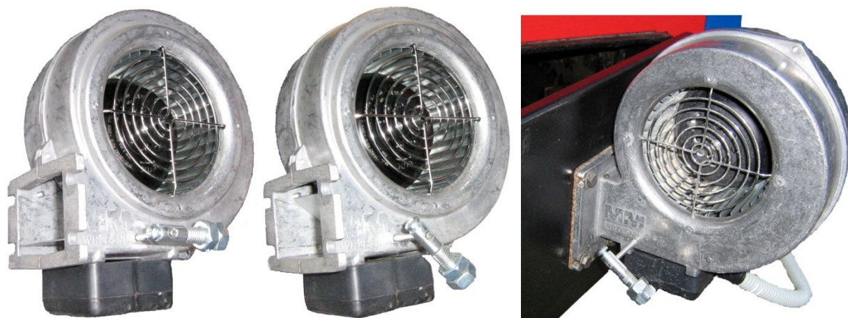
Рисунок 4 – Регулировка положения заслонки вентилятора
