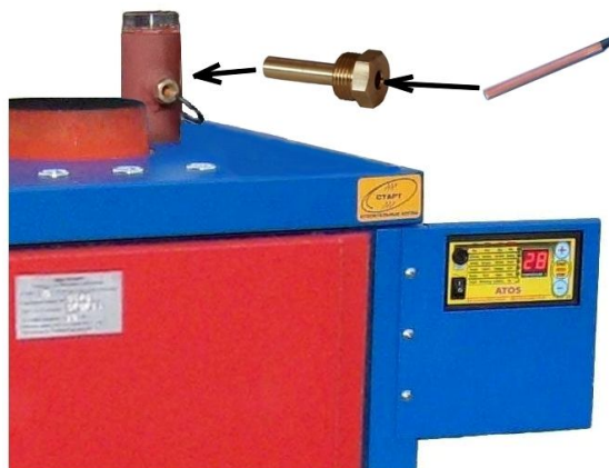
Рисунок 6 – Установка датчика температуры
