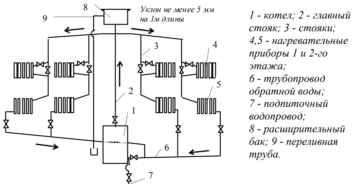
Рисунок 1 - Схема системы отопления
